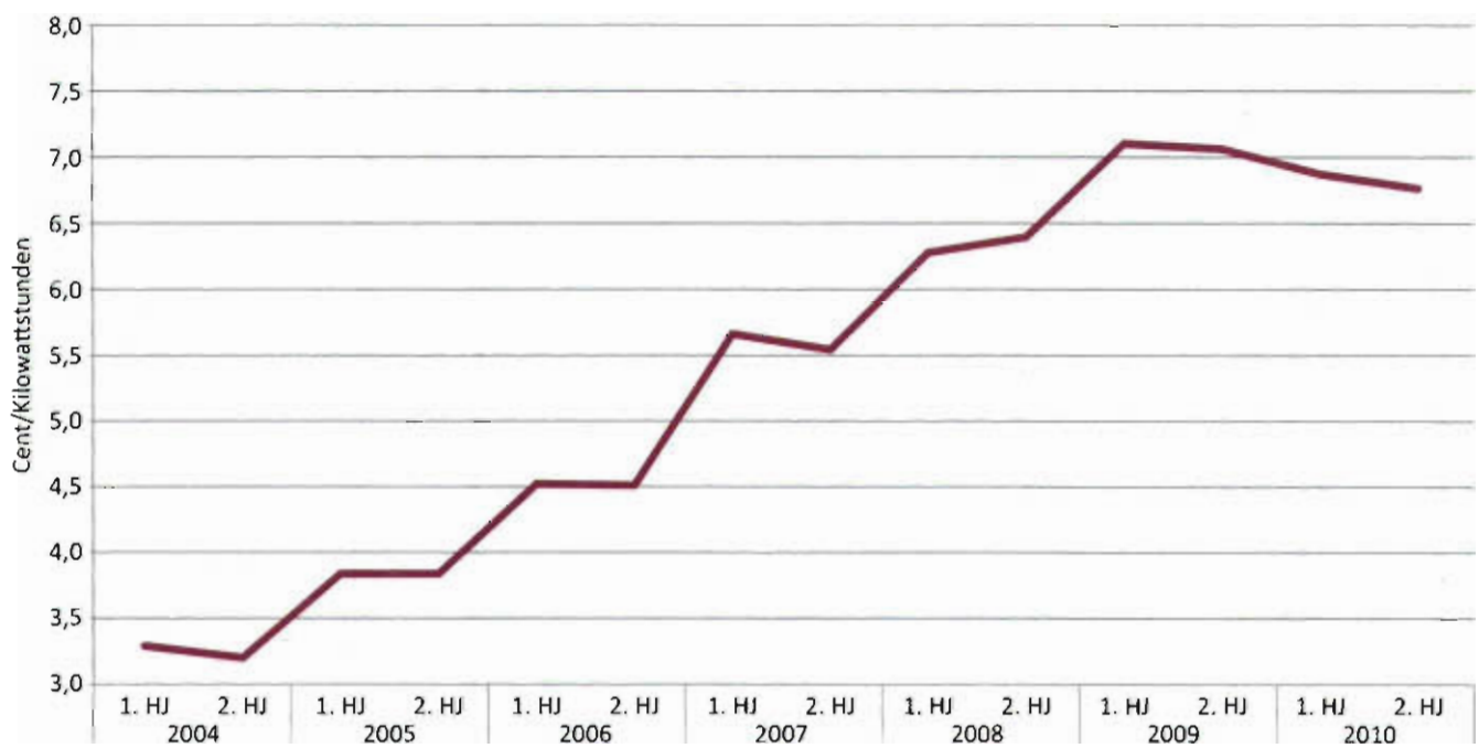
Abb. 3: Preisentwicklung Industriestrompreis
