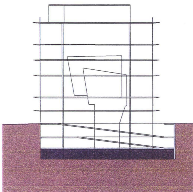
SCHNITT 1
