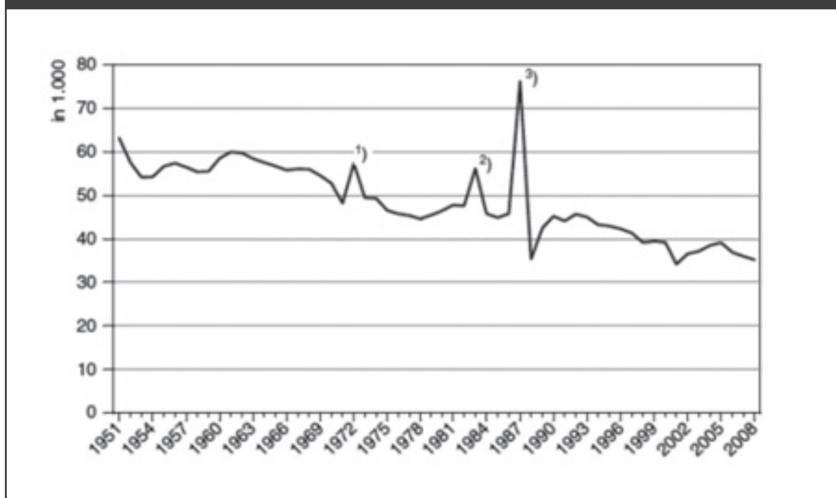
Grafik 19: Eheschließungen 1951 – 2008
