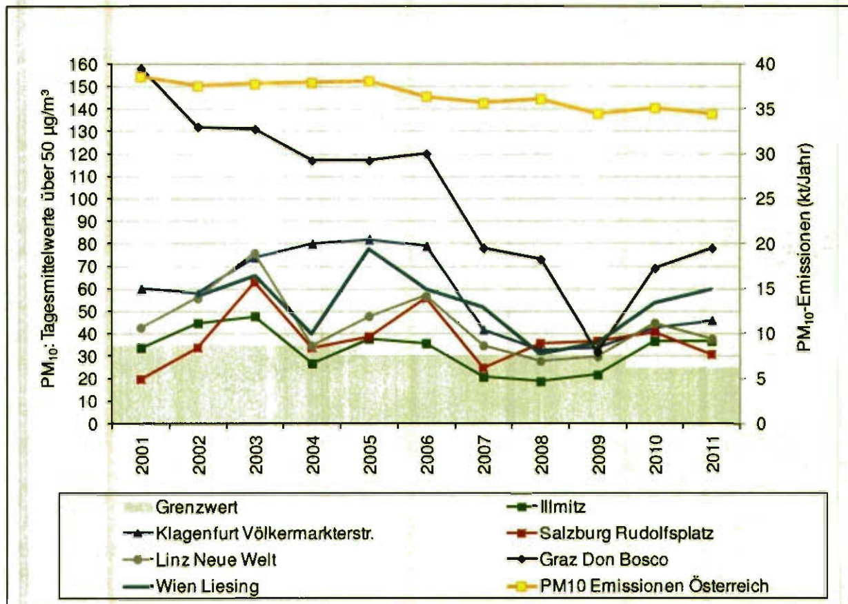
Abbildung 9: PM 10 – Anzahl der TMW über 50 µg/m 3 an ausgewählten Messstellen und PM 10 -Emissionen Österreichs, 2001–2011.
