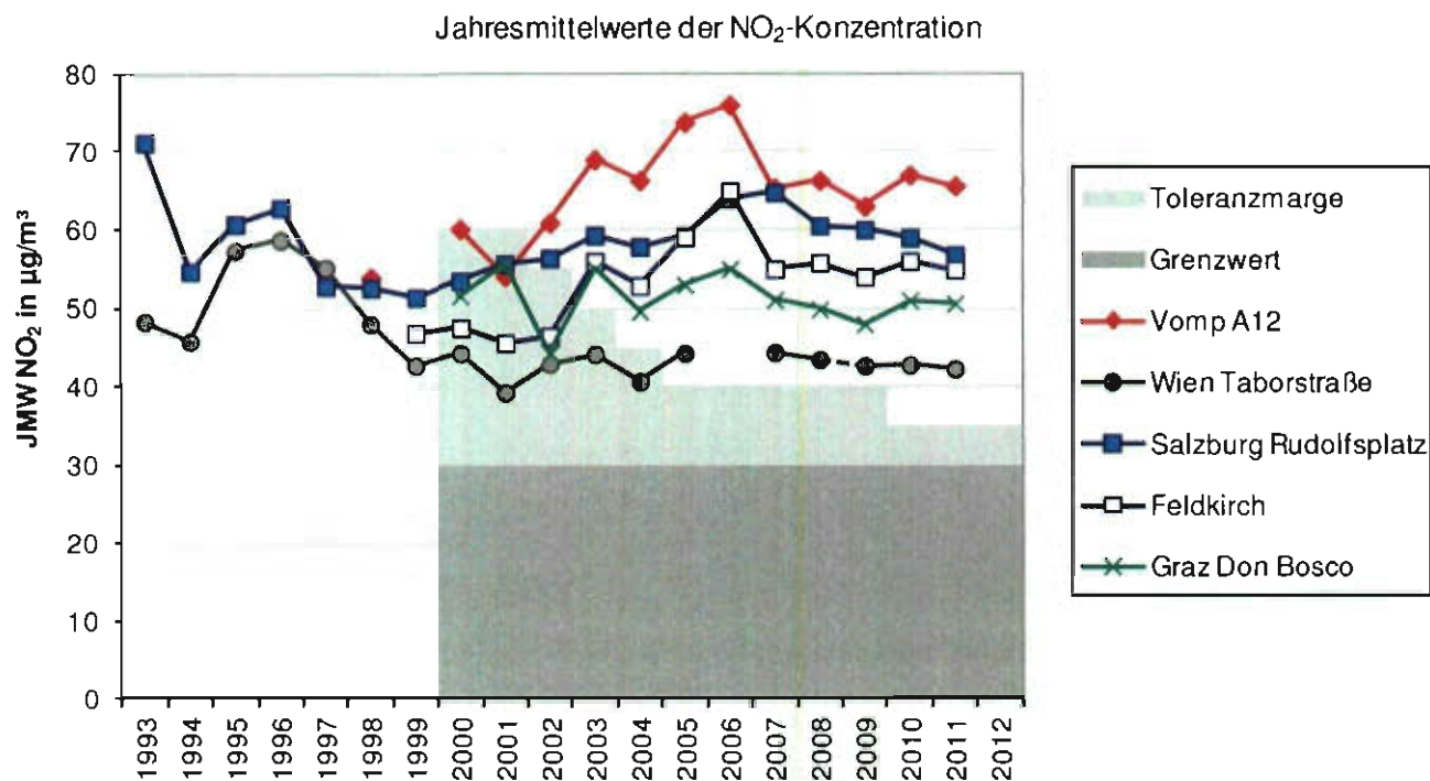
Abbildung 5: Jahresmittelwerte der NO 2 -Konzentration ausgewählter Stationen sowie zeitlicher Verlauf der Toleranzmarge für den Grenzwert des Jahresmittelwertes von NO 2 (Grenzwert ab 2000 in Kraft).
