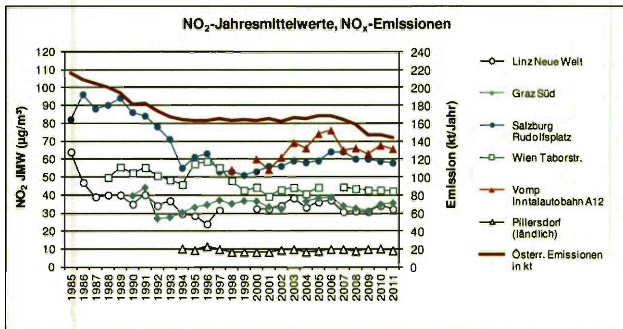
Abbildung 4: Jahresmittelwerte der \text{NO}_2 -Konzentration an hoch belasteten Messstellen und am Hintergrundstandort Pillersdorf sowie jährliche \text{NO}_x -Emissionen Österreichs 15 , 1985–2011.
