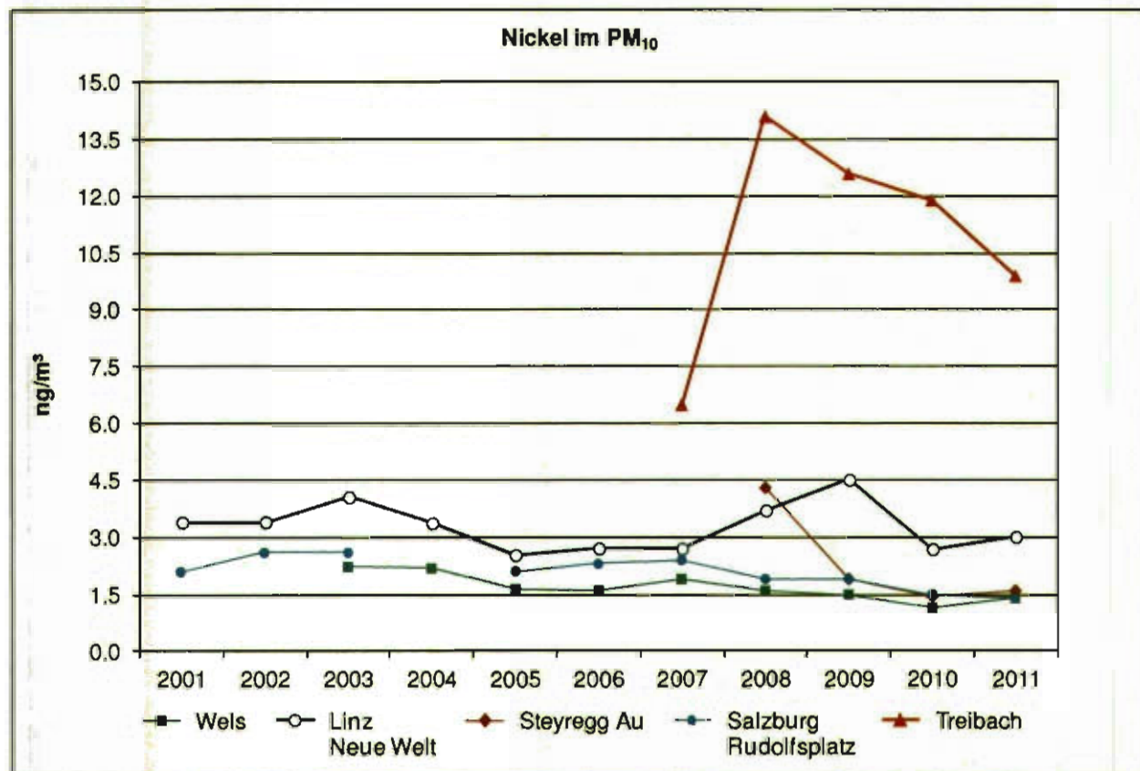
Abbildung 20: Trend der Konzentration von Nickel in PM 10 , 2001–2011.
