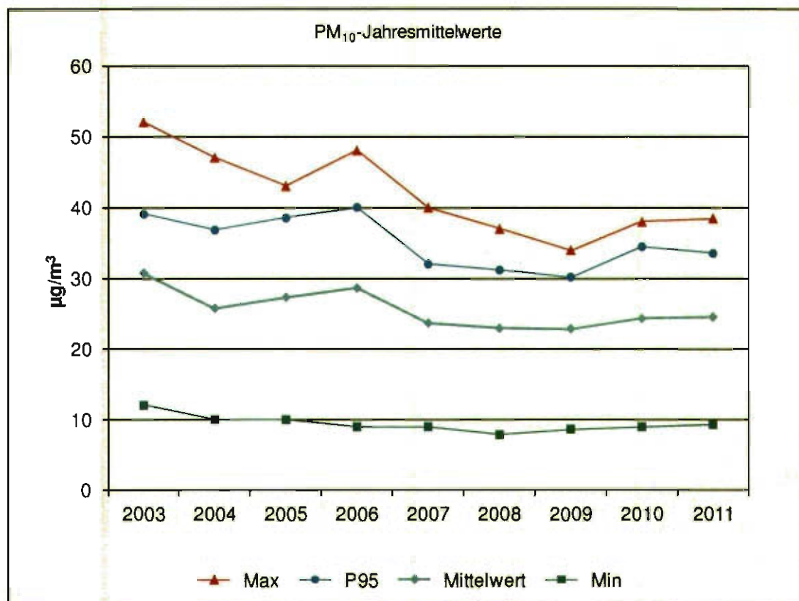
Abbildung 11: Maximum, 95-Perzentil, Mittelwert und Minimum der Jahresmittelwerte von PM_{10} an 69 durchgehend betriebenen PM_{10} -Messstellen in Österreich, 2003–2011.
