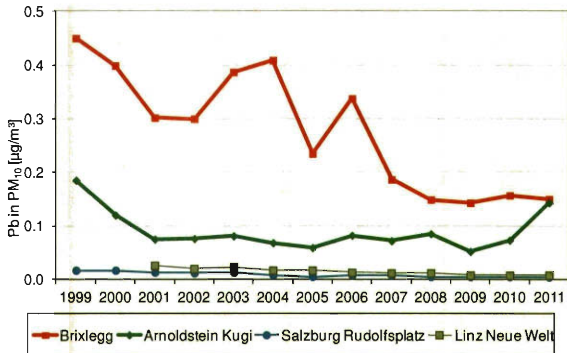
Abbildung 17: Jahresmittelwerte der Konzentration von Blei in PM_{10} , 1999–2011.
