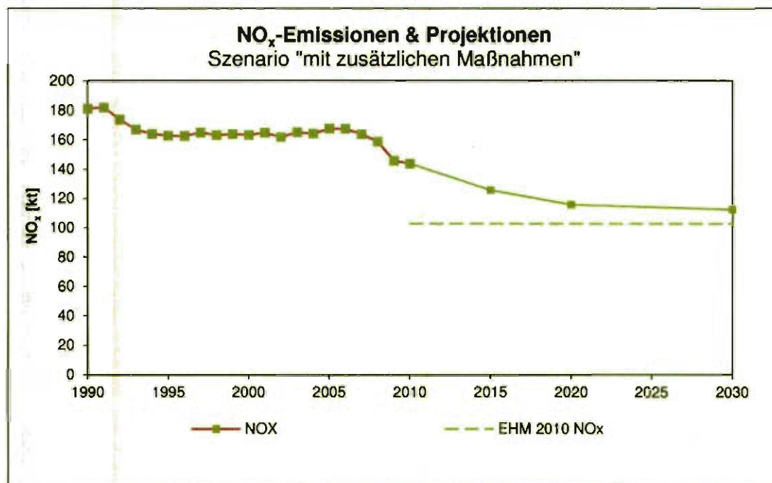
Abbildung 23: Emissionsprognose für NOx.
