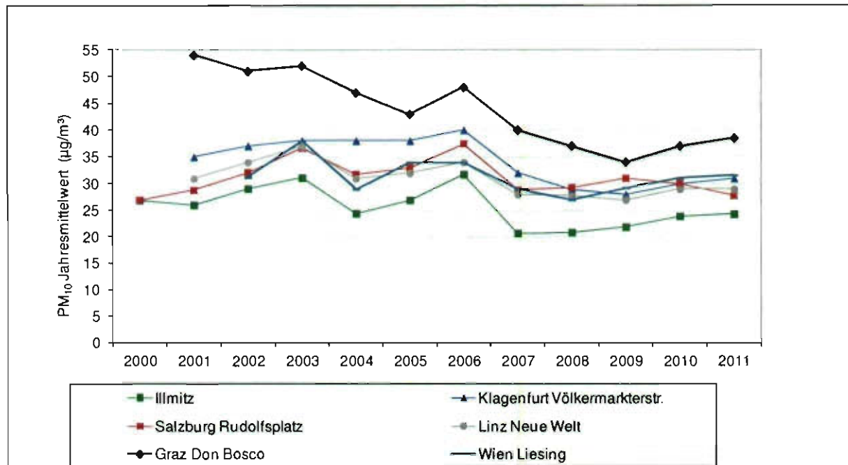
Abbildung 10: PM_{10} – Jahresmittelwerte an ausgewählten Messstellen, 2000–2011.
