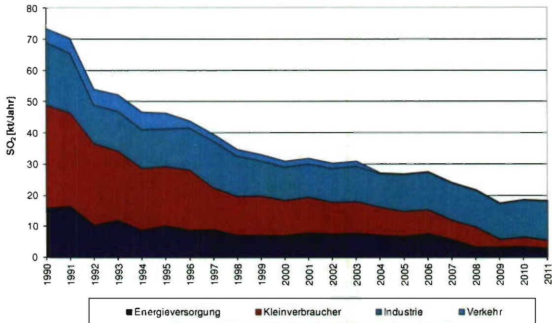
Abbildung 12: Trend der SO 2 -Emissionen in Österreich 1990–2011 (in kt/Jahr).
