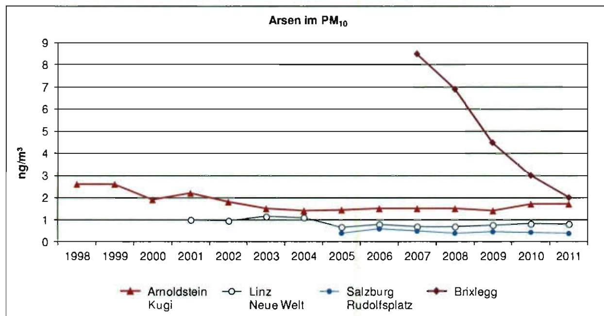
Abbildung 19: Trend der Konzentration von Arsen in PM 10 , 1998–2011.
