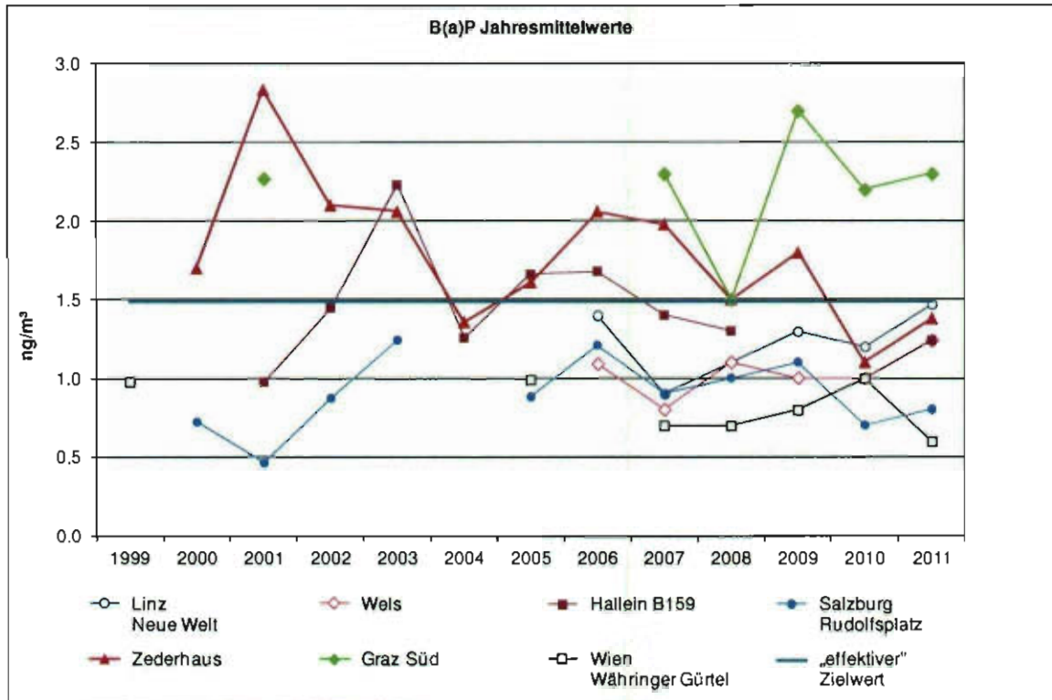
Abbildung 21: Trend der Benzo(a)pyren-Konzentration an ausgewählten Messstellen, 1999–2011 (JMWW).
