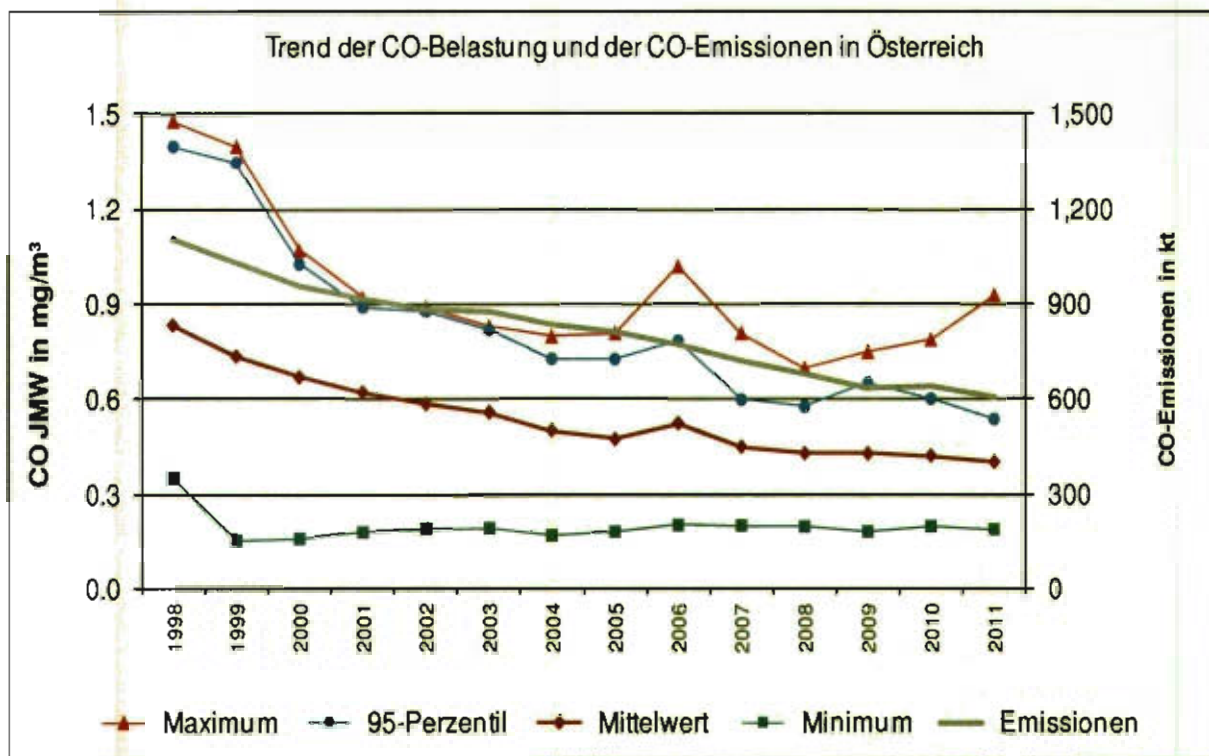
Abbildung 15: Maximum, 95-Perzentil, Mittelwert und Minimum der Jahresmittelwerte der CO-Konzentration an den 23 durchgehend betriebenen Messstellen 1998–2011 sowie CO-Emissionen in Österreich, 1998–2010.
