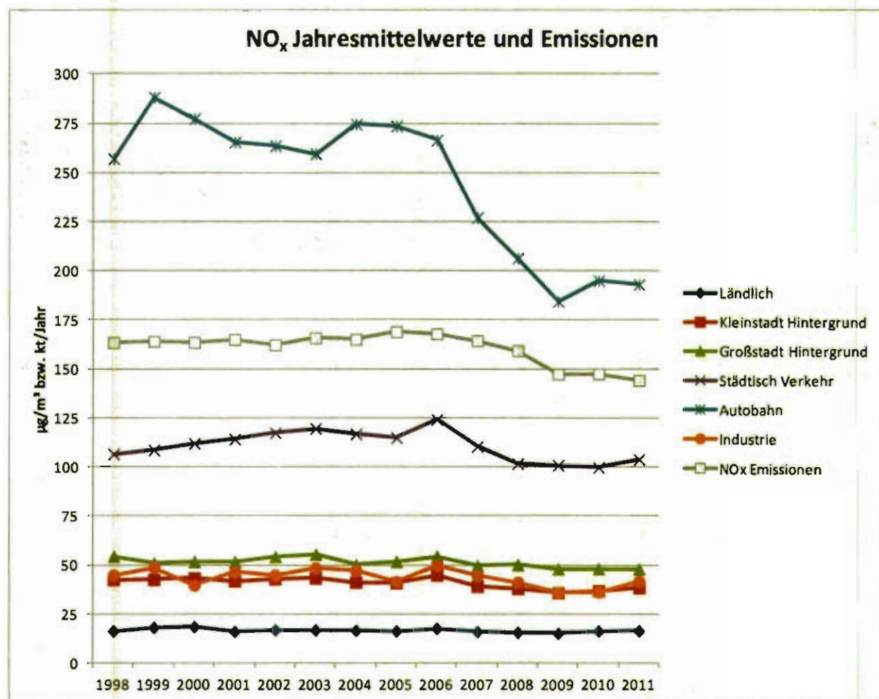
Abbildung 6: Mittelwert der \text{NO}_x -Konzentration über unterschiedliche Standorttypen, 1998–2011 (in \mu\text{g}/\text{m}^3 ), sowie \text{NO}_x -Emissionen Österreichs 1998–2010 (in \text{kt}/\text{Jahr} ).
