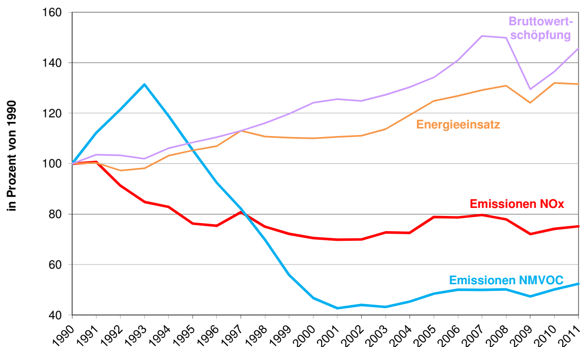
Abbildung 5.4: Emissionen stationärer Anlagen der Industrie 1990–2011, Energieverbrauch (Umwandlungseinsatz und Endverbrauch) und Bruttowertschöpfung (Daten: Umweltbundesamt, Statistik Österreich)
