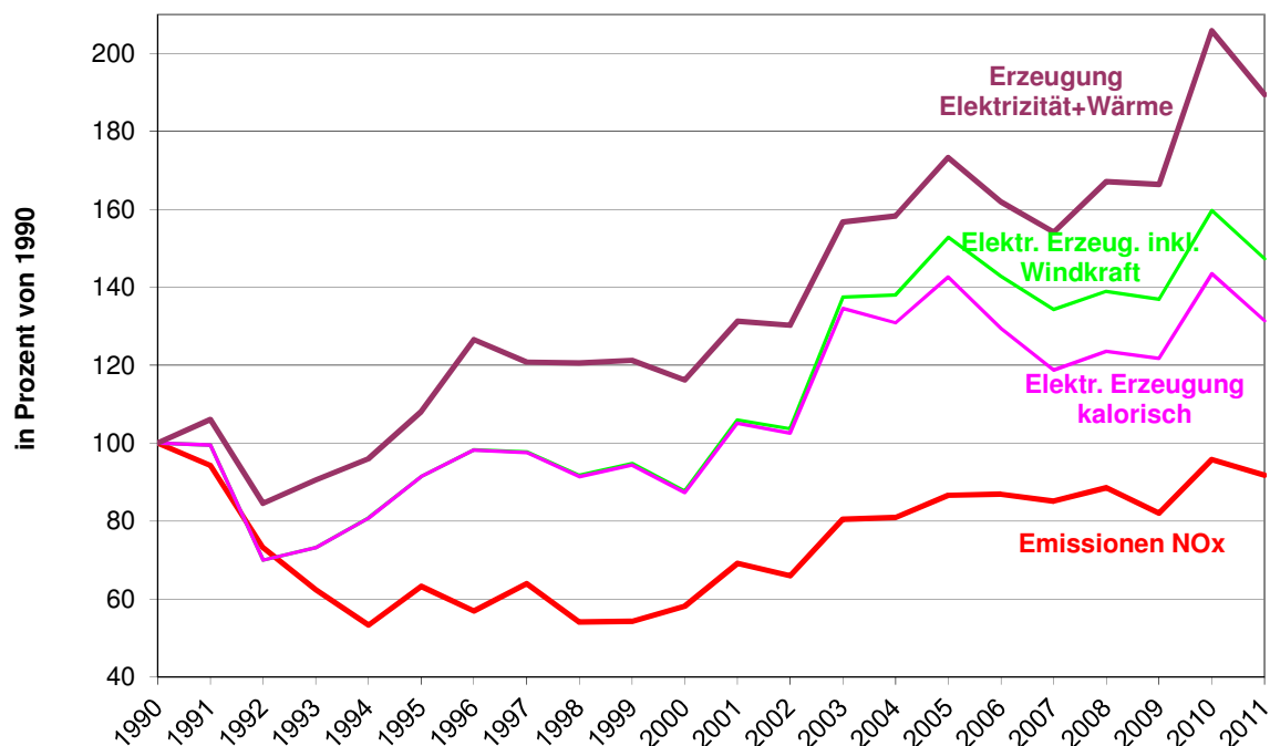
Abbildung 5.1: Öffentliche Energieversorgung 1990–2011 – NO x -Emissionen, Erzeugung von elektrischer Energie aus kalorischen Kraftwerken und Windkraft sowie von Elektrizität plus Wärme (Umwandlungsausstoß) (Daten: Umweltbundesamt, Statistik Österreich)
