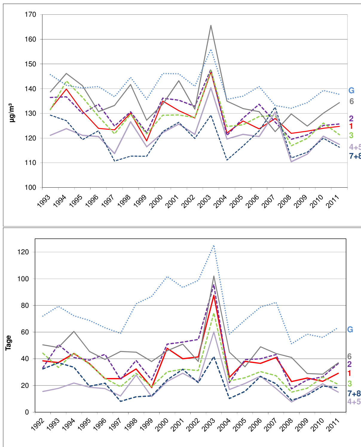
Abbildung 3.4 – Oben: 98-Perzentil der Einstundenmittelwerte in den Jahren 1993–2011 nach Ozon-Überwachungsgebieten. Unten: Anzahl der Tage mit Überschreitung des langfristigen Zieles zum Schutz der menschlichen Gesundheit ( \text{MW}_8 > 120 \mu\text{g}/\text{m}^3 ) pro Jahr in den Ozon-Überwachungsgebieten als Mittelwert der Stationen im jeweiligen Gebiet 1992–2011. (Ozon-Überwachungsgebiete „1“ bis „8“; G = Gebirge, d.h. Messstellen über 1.500 m Seehöhe)
