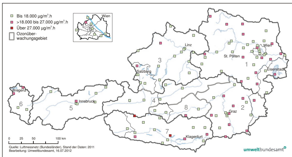
Abbildung 3.2: AOT40-Werte (Mai–Juli, 08:00–20:00 Uhr), Mittel über den Zeitraum 2007–2011 (Höher als 18.000 \mu\text{g}/\text{m}^3 \cdot \text{h} = Überschreitung des Zielwertes)
