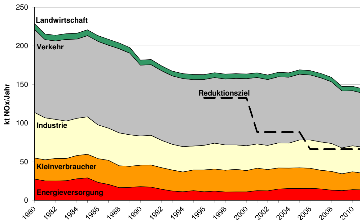
Abbildung 4.2: \text{NO}_x -Emissionen 1980–2011 und ozongesetzliches Reduktionsziel
