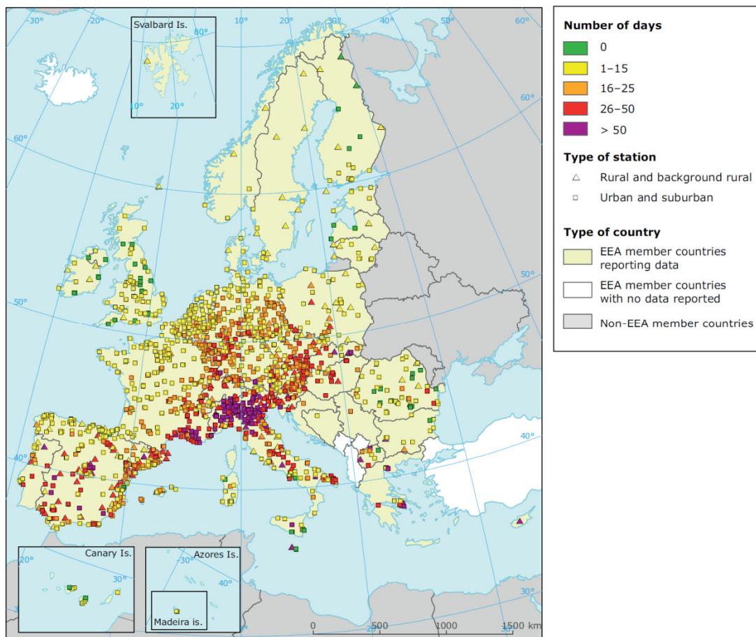
Abbildung 3.6: Jährliche Überschreitung des langfristigen Zieles zum Schutz der menschlichen Gesundheit für den Mittelungszeitraum 2009–2011 (Überschreitung an mehr als 25 Tagen = Überschreitung des Zielwerts) (Grafik: EEA 4 )
