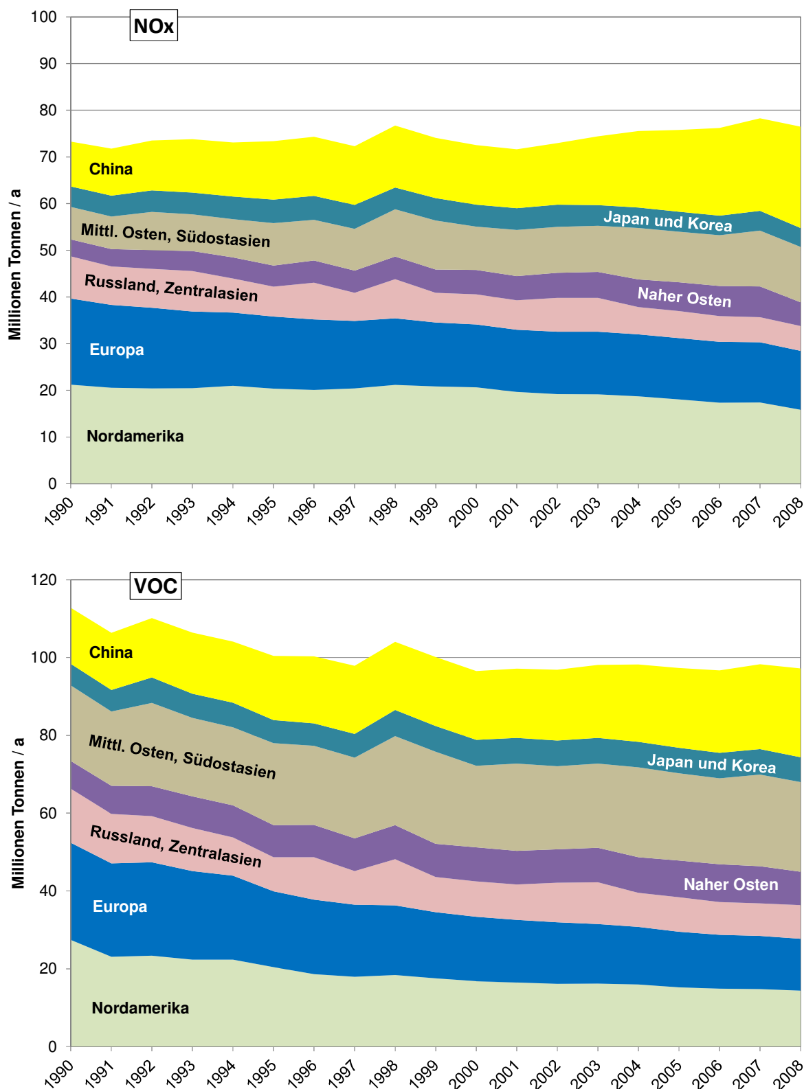
Abbildung 4.5: Entwicklung der anthropogenen Emissionen von NOx und VOC 1990–2008 in Europa, Nordamerika und Asien (Quelle: EDGAR 16 )
