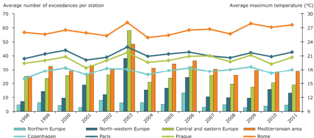
Abbildung 3.5: Mittlere Anzahl der Tage mit Überschreitung des langfristigen Zieles zum Schutz der menschlichen Gesundheit ( MW_8 > 120 \mu\text{g}/\text{m}^3 ) pro Messstation in den Regionen Europas 1998–2011 (in \mu\text{g}/\text{m}^3 ) und Temperaturen in ausgewählten Städten (Grafik: EEA 4 )
