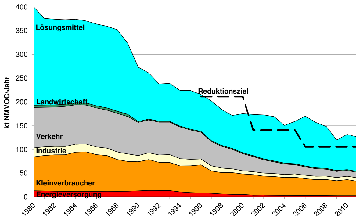
Abbildung 4.4: NMVOC-Emissionen 1980–2011 und ozongesetzliches Reduktionsziel
