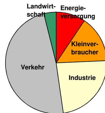
Abbildung 4.1: NO x -Emissionen 2011
