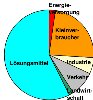
Abbildung 4.3: NMVOC-Emissionen 2011 nach Sektoren
