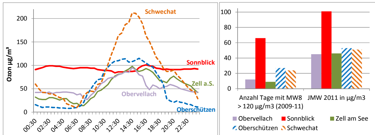
Abbildung 3.7: Ozonebelastung am Hohen Sonnblick im Vergleich zu benachbarten Stationen in inneralpinen Tallagen und zu Stationen am Rande Wiens und im Südburgenland. Links: Exemplarischer Tagesverlauf an einem stark belasteten Tag (August 2011). Rechts: Anzahl der Tage mit max. MW8 > 120 \mu\text{g}/\text{m}^3 im Mittel 2009–2011 und Ozonejahresmittelwerte 2011
