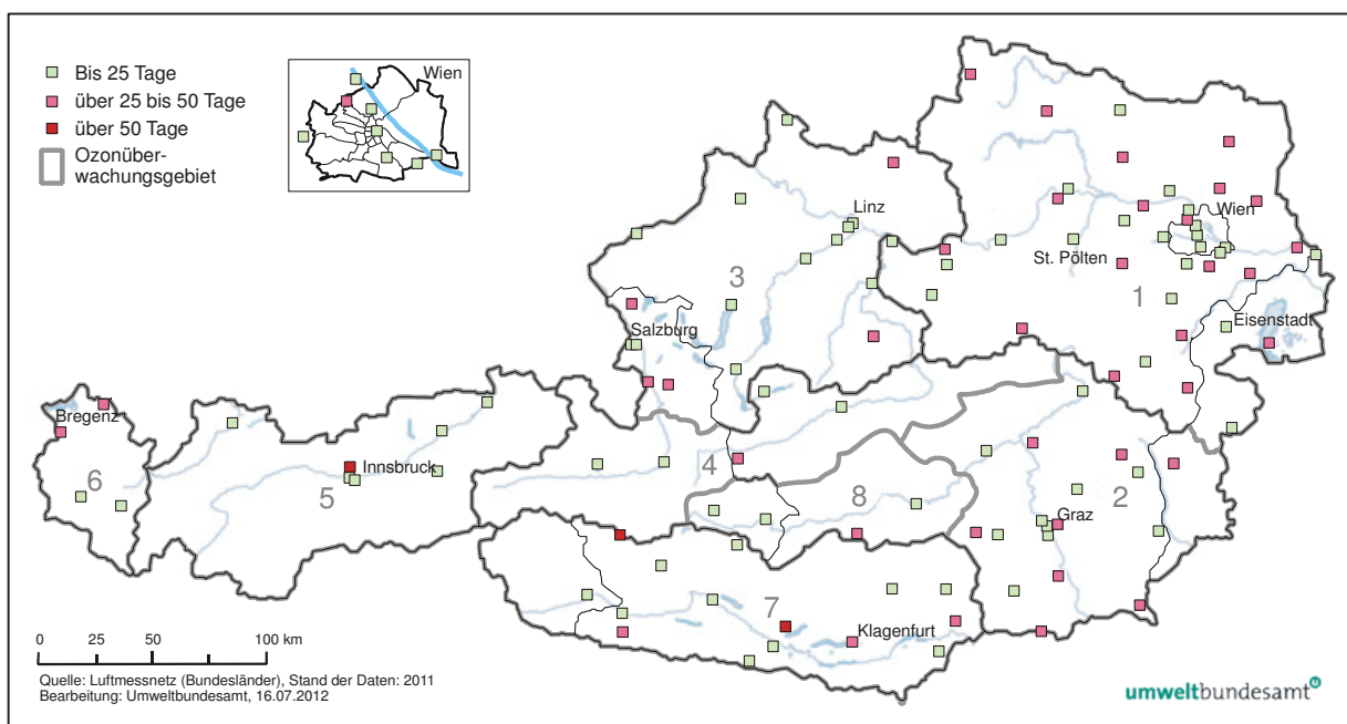
Abbildung 3.1: Jährliche Überschreitung des langfristigen Ziels zum Schutz der menschlichen Gesundheit für den Mittelungszeitraum 2009–2011 (Überschreitung an mehr als 25 Tagen = Überschreitung des Zielwerts)
