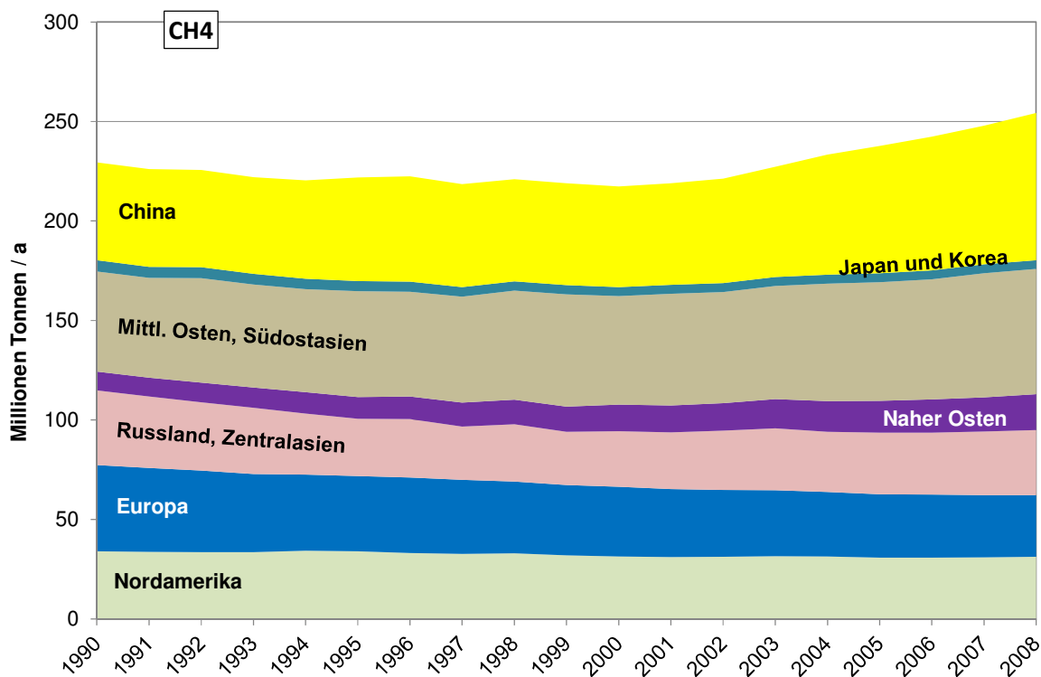
Abbildung 4.6: Entwicklung der anthropogenen Emissionen von Kohlenmonoxid und Methan 1990–2008 in Europa, Nordamerika und Asien (Quelle: EDGAR 16 )
