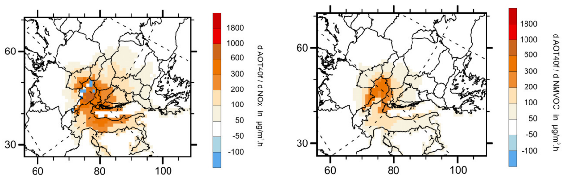
Abbildung 3.8: Modellierter Rückgang der Ozonebelastung als AOT40 in Österreich und benachbarten Ländern bei einer 15%-igen Emissionsreduktion in Österreich für \text{NO}_x (links) bzw. NMVOC (rechts). Positive Werte = Rückgang, negative Werte = Anstieg. (MSC-W Data Note 1/2012) 6
