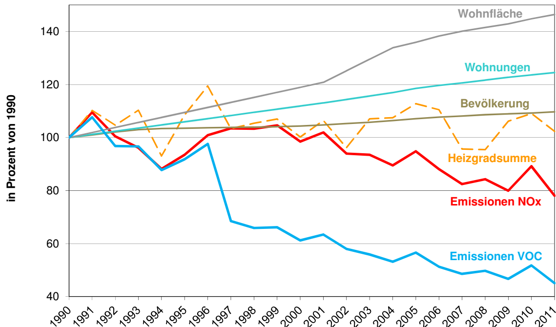
Abbildung 5.2: Hausheizungen 1990–2011 – NO x -Emissionen im Vergleich zu Bevölkerung, Zahl der Wohnungen (Hauptwohnsitze) und deren Gesamtfläche (Daten: Umweltbundesamt, Statistik Österreich)
